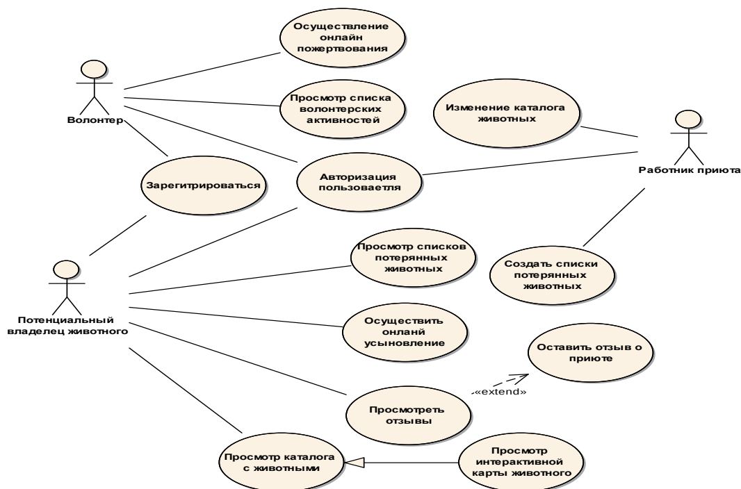
Рисунок 1- Диаграмма вариантов использования web-приложения
