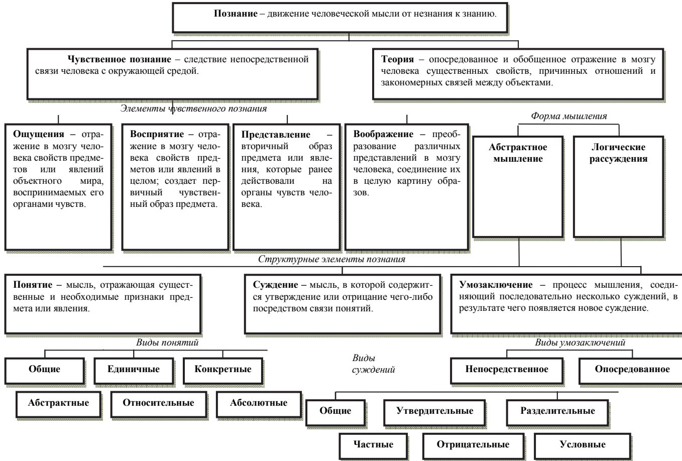
Рис. 1.3. Структурная схема процесса познания
