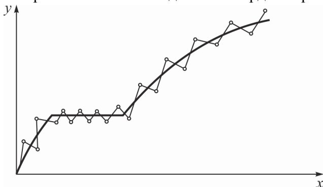
Рис. 5.2. Скачкообразное изменение функции
