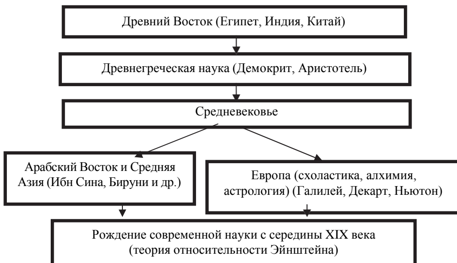
Рис. 1.2. Этапы развития науки
