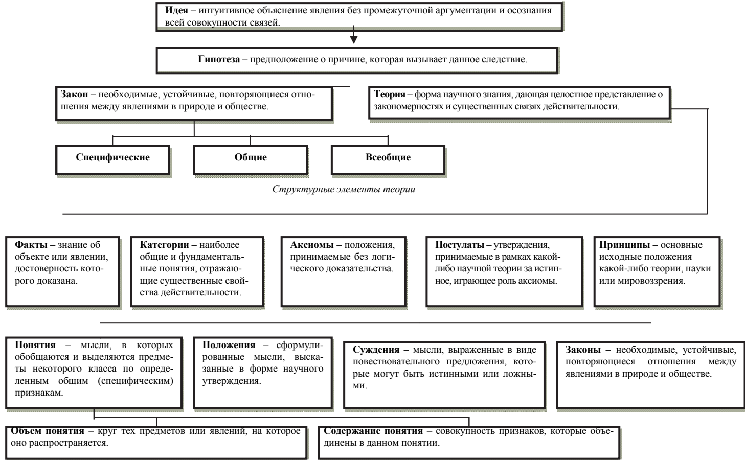
Рис. 1.4. Основные структурные элементы теории познания
