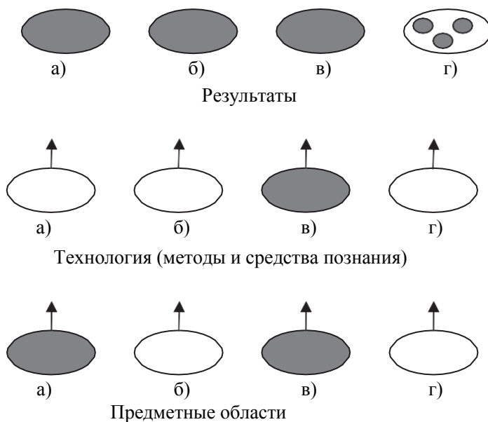
Рис. 2.3. Варианты получения новых научных результатов
