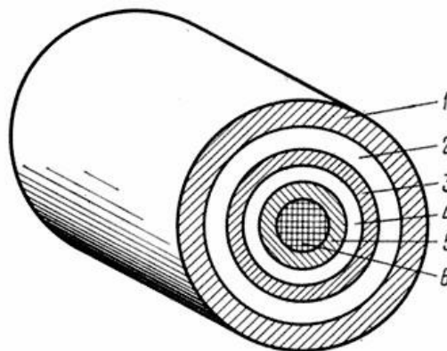
Рис. 5.11. Ядерный термоэмиссионный преобразователь: 1 – защита; 2 – охладитель; 3 – анод; 4 – вакуум;
