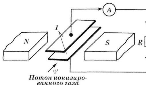
Рис. 5.5. Принцип работы МГД-генератора
