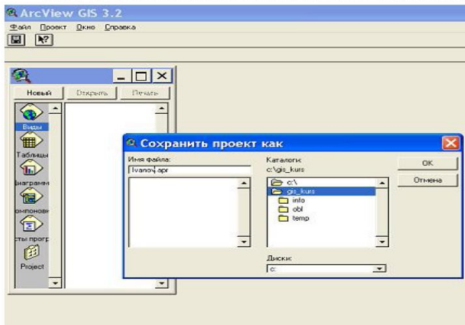
Рис.2. Сохранение проекта
