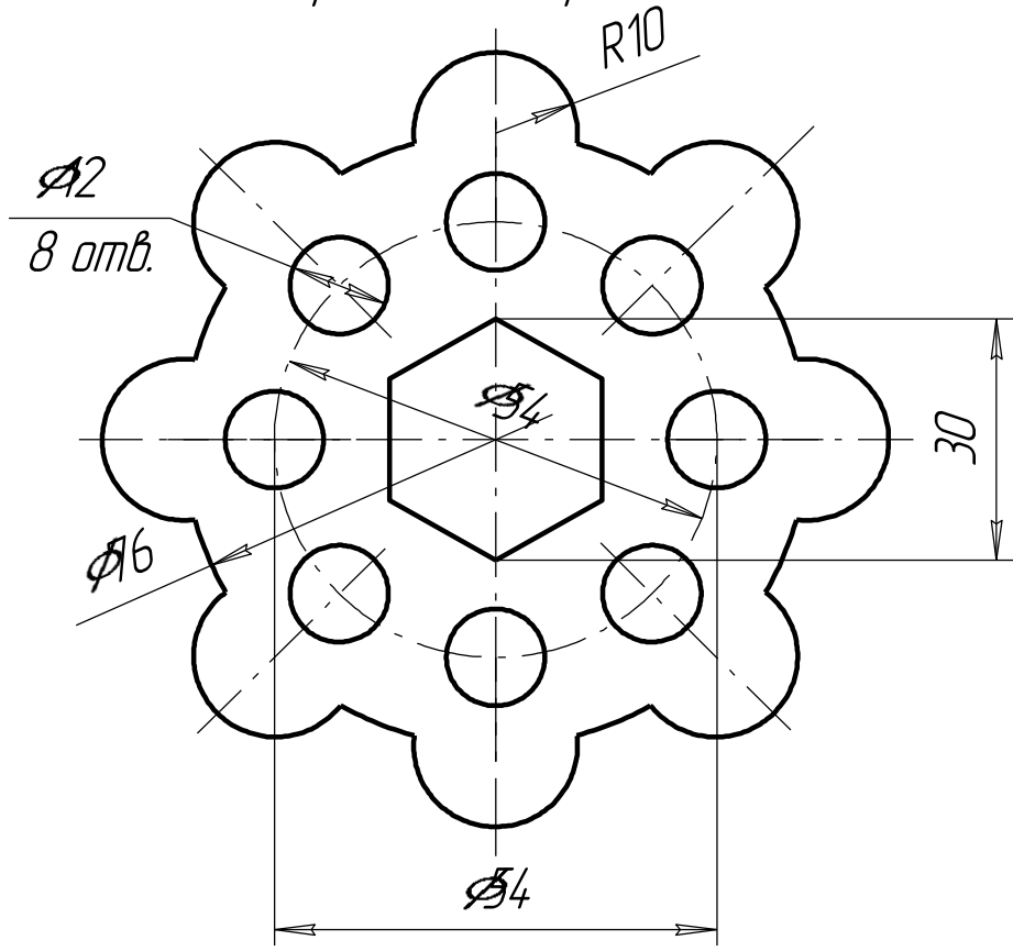
Вариант №9 Крышка
