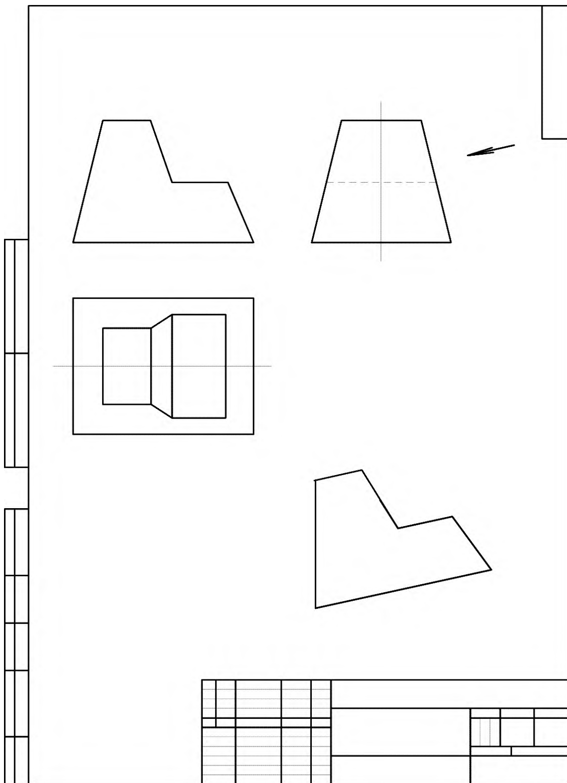
Рис. 1.28 Пример выполнения задания «Построение видов».
