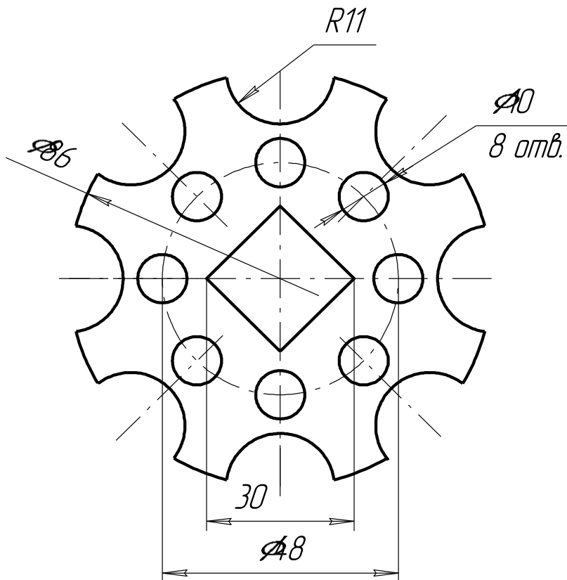
Вариант №8 Крышка
