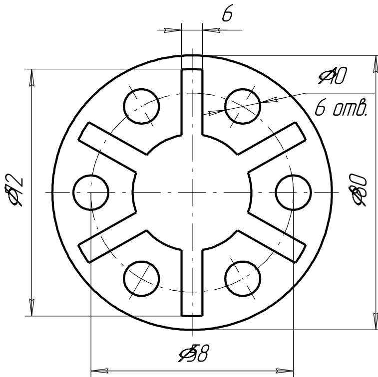
Вариант №7 Крышка
