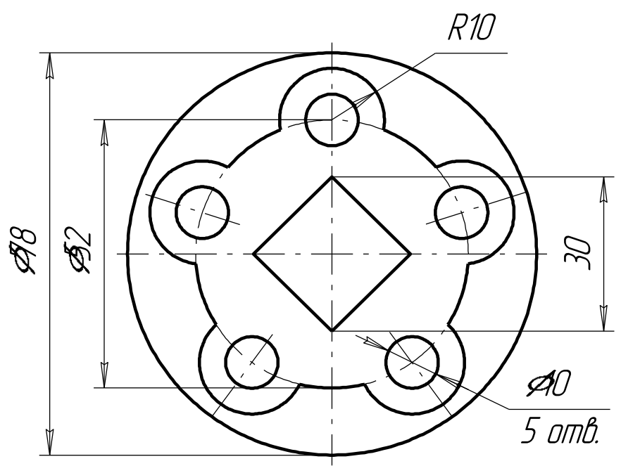
Вариант №10 Крышка
