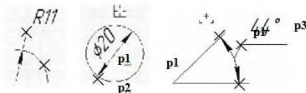
Рис. 2.10. Нанесение размеров дуги, диаметра окружности и углового разме-
