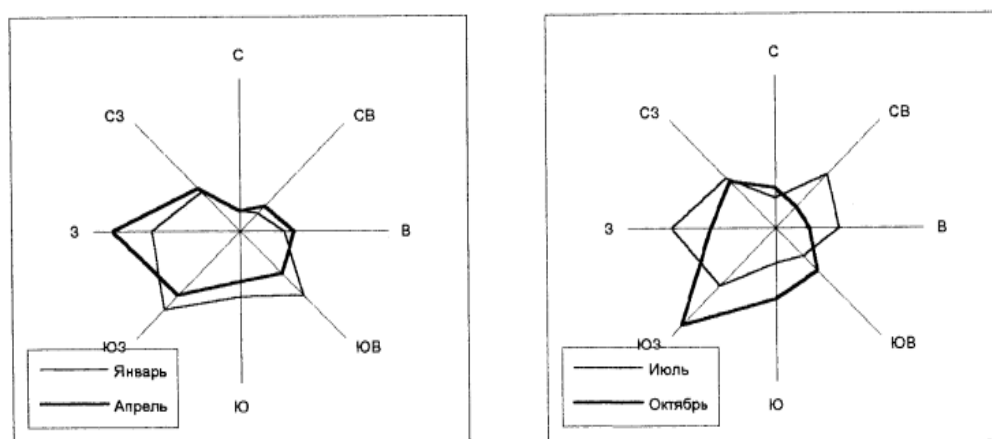
Рис.8. Розы ветров для характерных месяцев года южного побережья Финского залива
