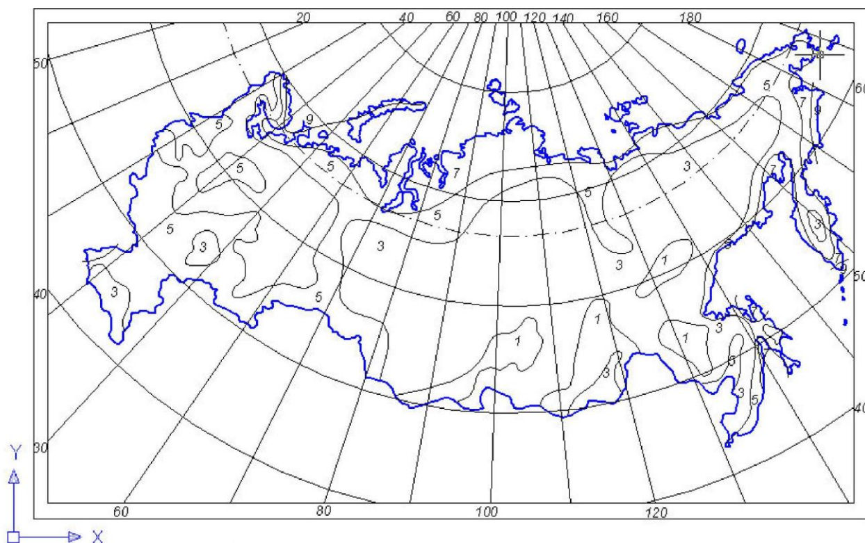
Рис.11. Параметр масштаба \beta функции Вейбулла (м/с). Год
