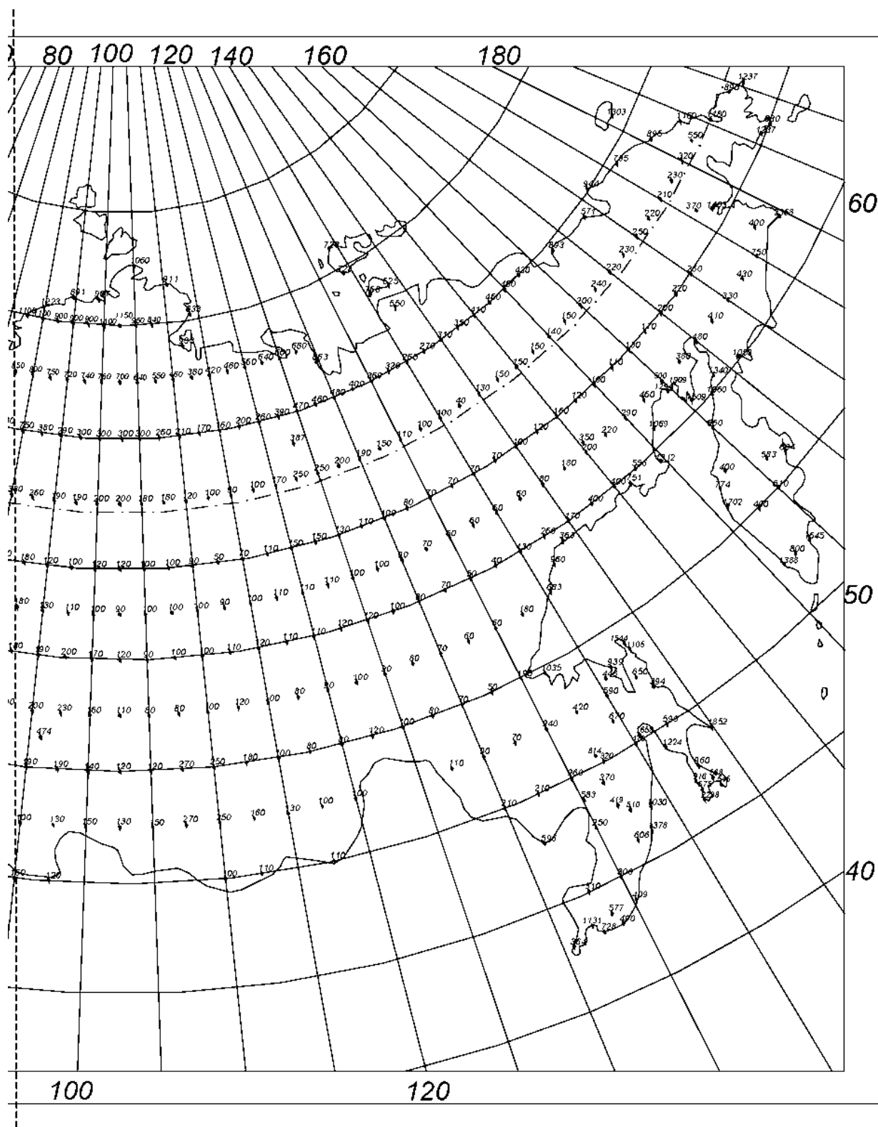
Рис.3. Природные потенциальные ветроэнергетические ресурсы России (Вт/м) (правая часть)
