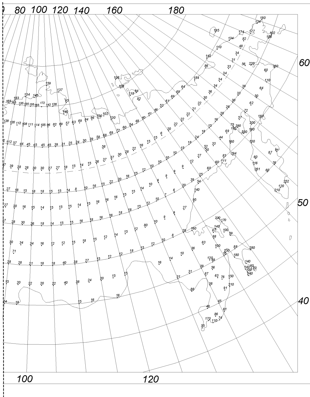
Рис.4.Плотность технического ветроэнергетического потенциала (H=50м) (правая часть)
