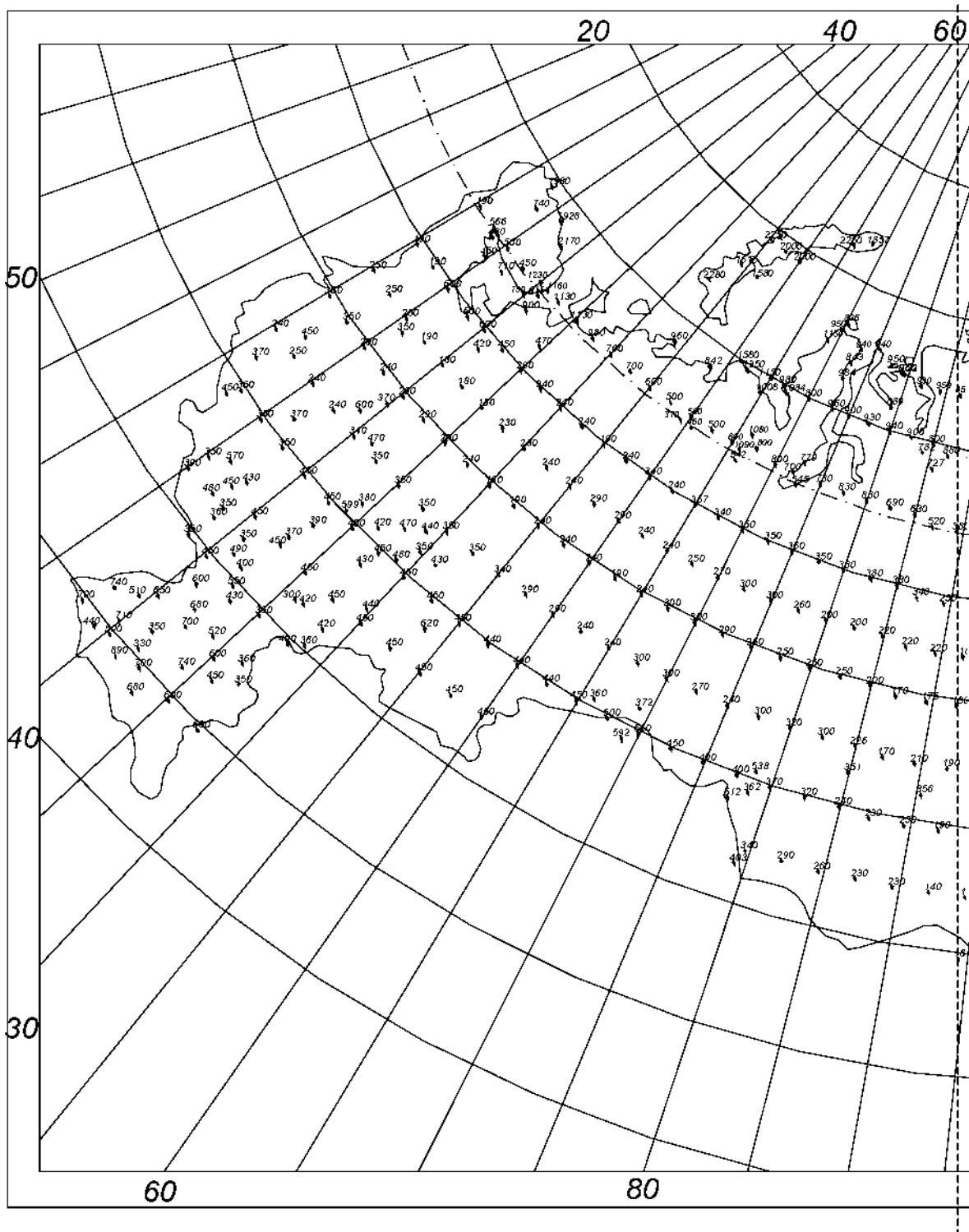
Рис.3. Природные потенциальные ветроэнергетические ресурсы России (Вт/м) (левая часть)
