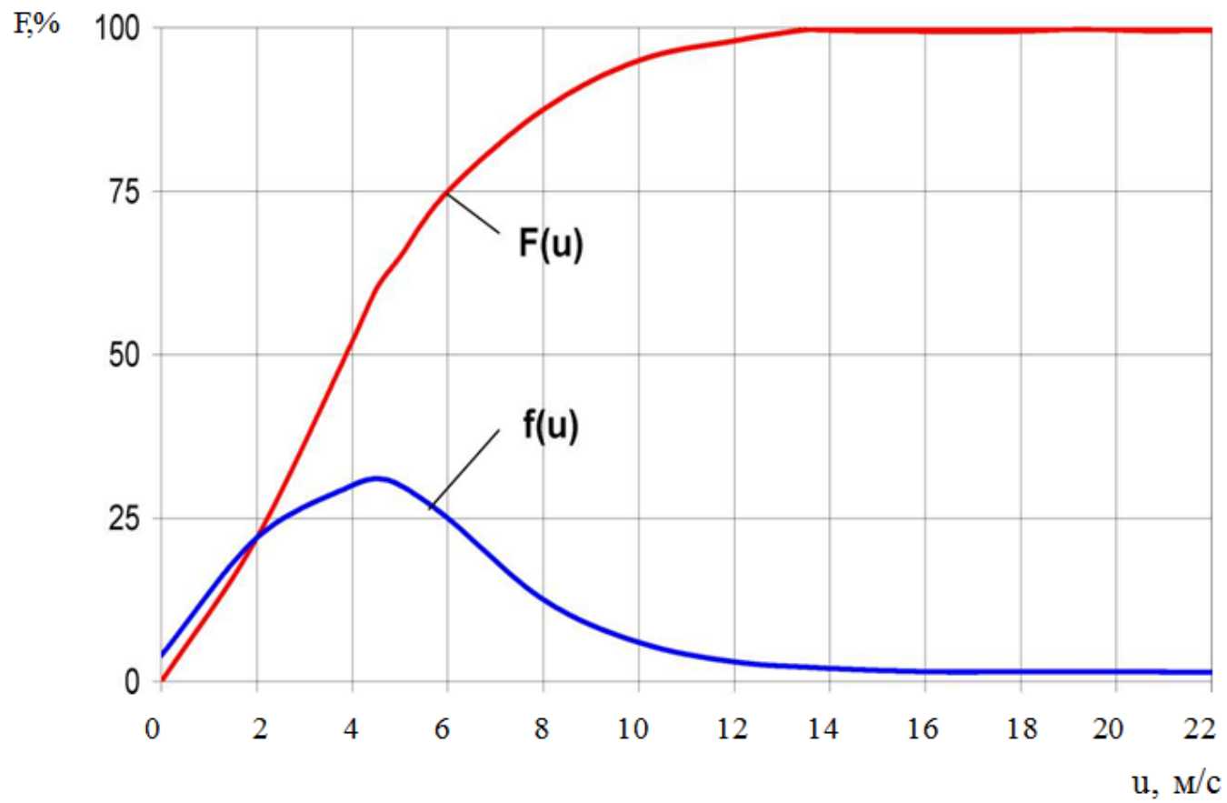
Рис.10. Интегральная F(u) и дифференциальная f(u) повторяемости скорости ветра (станция Ломоносов)
