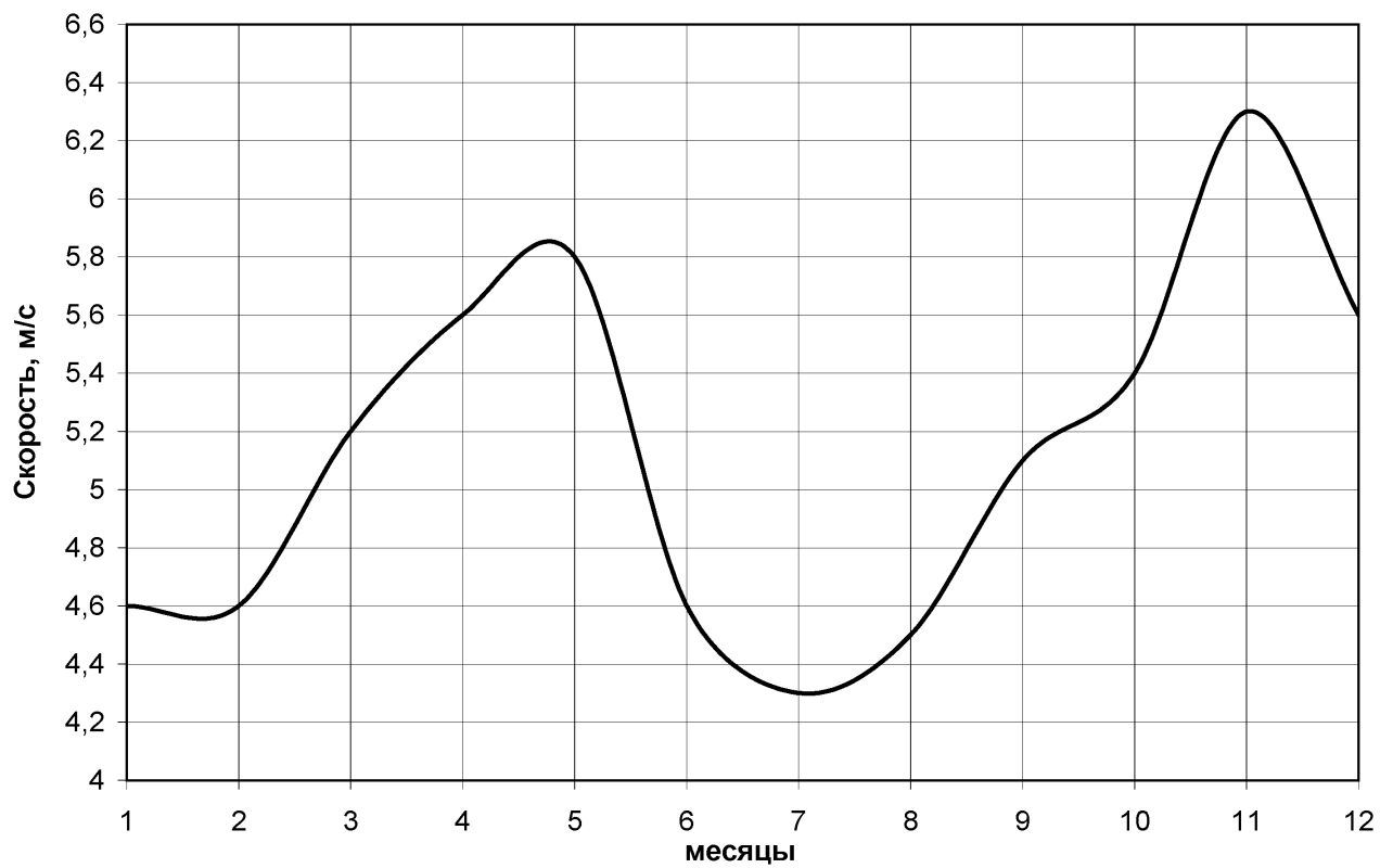
Рис.6. Годовой ход скорости ветра, г. Хабаровск
