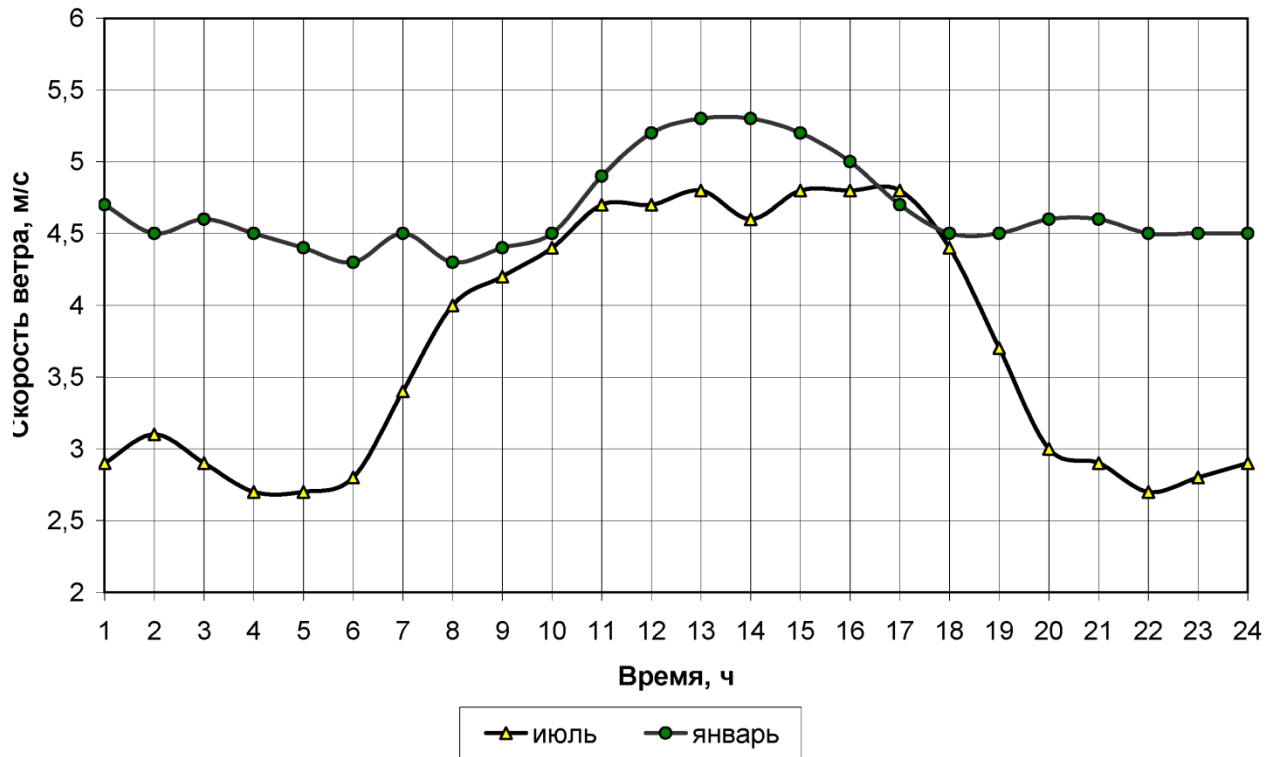
Рис.5. Суточный ход скорости ветра в г. Хабаровске.
