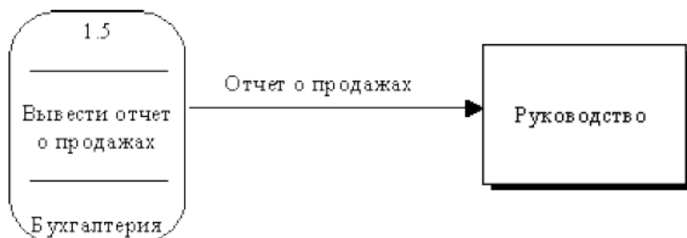
Рис. 4.38. Поток данных
