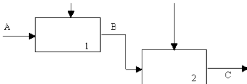
Рис. 4.8. Последовательная связность
