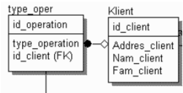
Рис. 4.33 Неидентифицирующая связь
