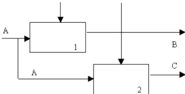
Рис. 4.7. Коммуникационная связность
