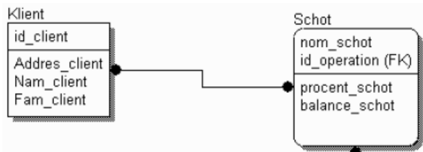
Рис. 4.34. Связь «многие-ко-многим»
