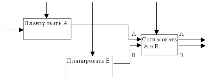
Рис. 4.6. Процедурная связность
