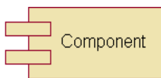
Рис. 3.6. Диаграмма компонентов.
