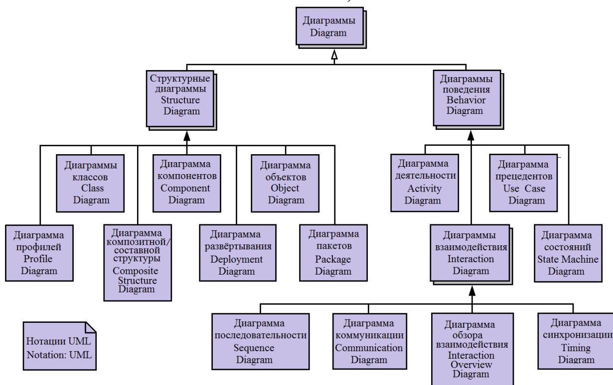
Рис. 3.4. Структура диаграмм.
