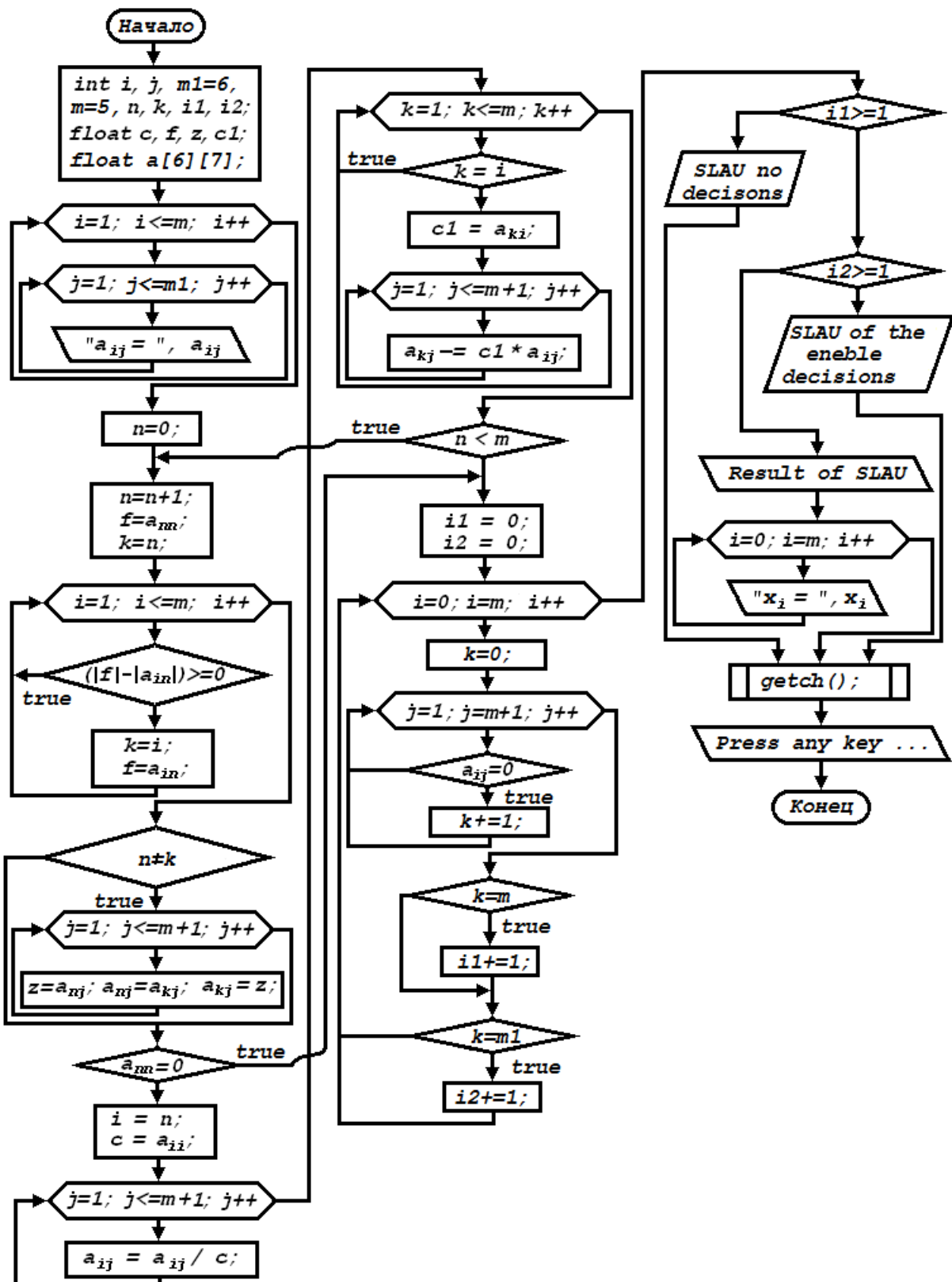
Рис.5.15. Детальная схема блок-схема алгоритма метода Жордана-Гаусса.
