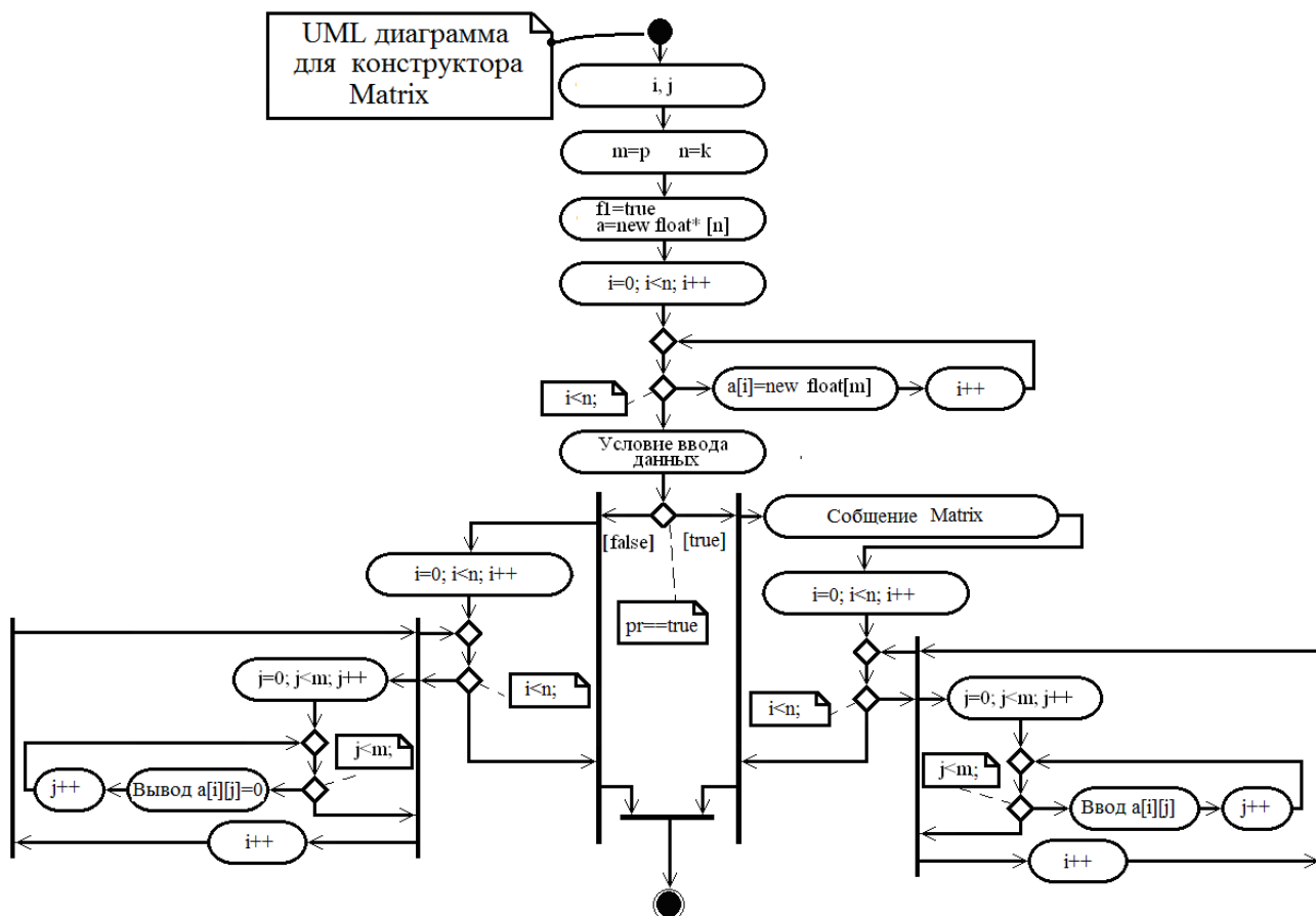
Рис.6. 24. UML – диаграмма конструктора класса matrix.
