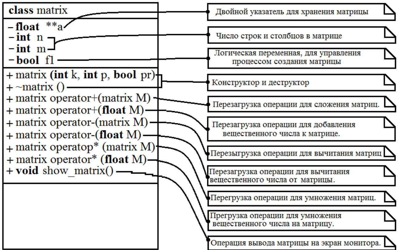
Рис.6.22. Класс matrix .
