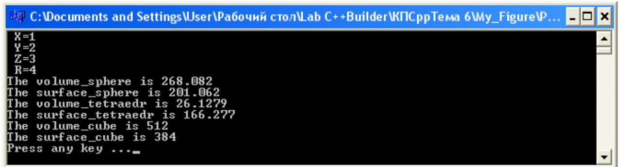
Рис.6.12. Поверхности и объемы фигур при заданных координатах.
