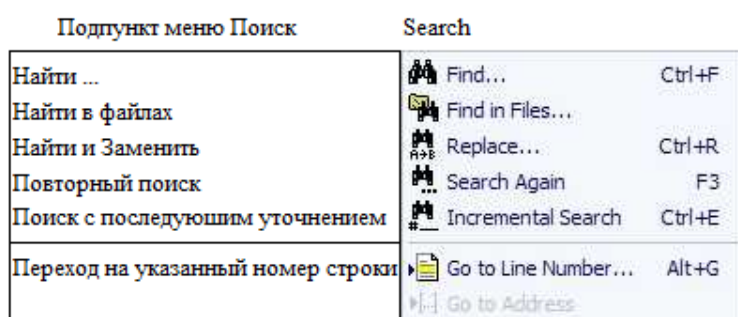
Рис. 1.7. Поисковые операции.
