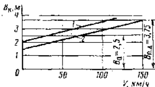
Рис. 8.7. Зависимость ширины коридора B_k движения от скорости движения транспортных средств:
