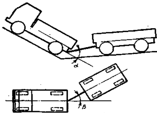
Рис. 8.4. Углы гибкости автопоезда в вертикальной и горизонтальной плоскостях
