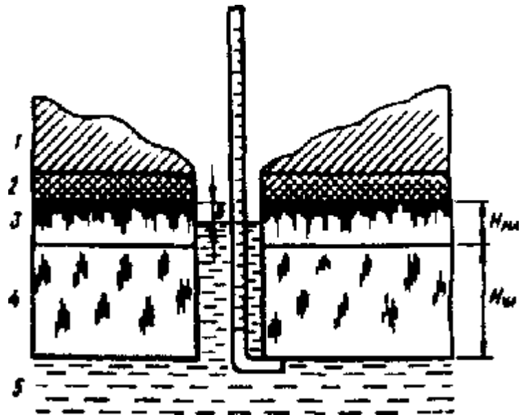
Рис. 6.6. Измерение толщины льда: 1 – снег; 2, 3 и 4 – соответственно снеговой, мутный и чистый лед; 5 – вода; 6 – уровень воды в лунке, равный 0,1 (H_{ч.л} + H_{м.л})
