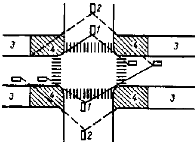
Рис. 6.4. Видимость на перекрестке при наличии снежных валов: 1 и 2 – видимость соответственно при несрезанном и частично срезанном вале; 3 – снежный вал; 4 – участки частичного удаления вала
