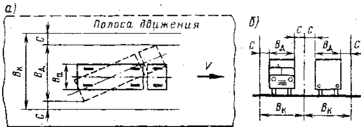
Рис. 8.6. Коридор движения: а – на однополосной дороге; б – на двухполосной дороге; B_a – статическая ширина автомобиля; B_d – динамическая ширина автомобиля; B_k – коридор движения; C – зазоры безопасности
