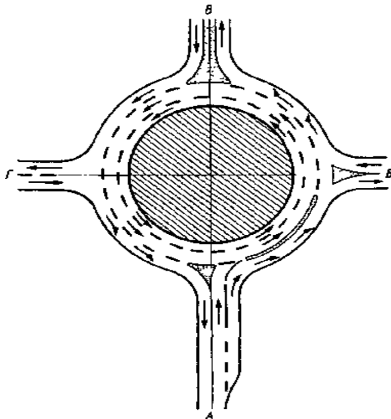
Рис. 5.10. Круговая развязка с примерами канализирования движе- ния
