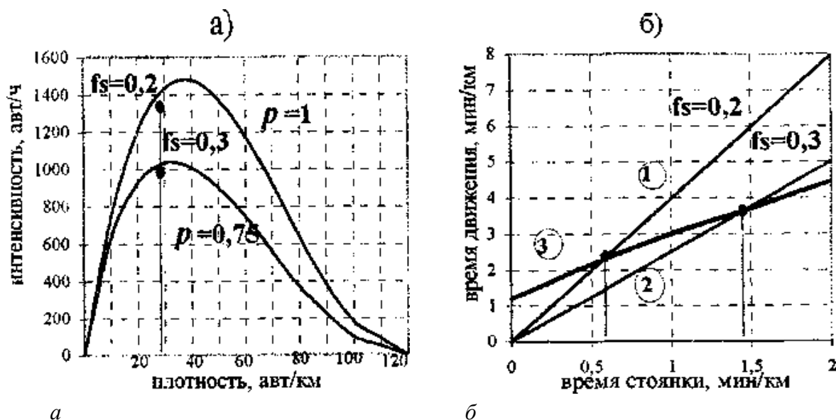
Рис.3.9. Основная диаграмма транспортного потока (а) и зависимость между временем движения и временем стоянки (б): 1 – линия постоянного значения доли стоящих автомобилей для f_s = 0,2 ; 2 – линия постоянного значения доли стоящих автомобилей для f_s = 0,3 ; 3 – зависимость между временем движения и временем стоянки
