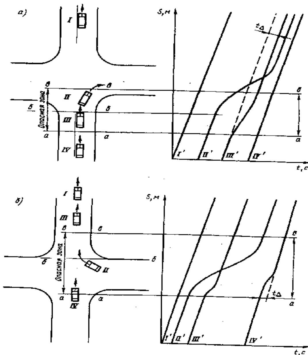
Рис. 5.3. Схема движения при маневрах:
