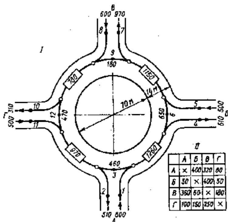
Рис.5.9.Результатыисследованиятран- спортныхпотоконаразвязкескруговым движением (I) и матрица транспортныхкорреспонде- нций(II)
