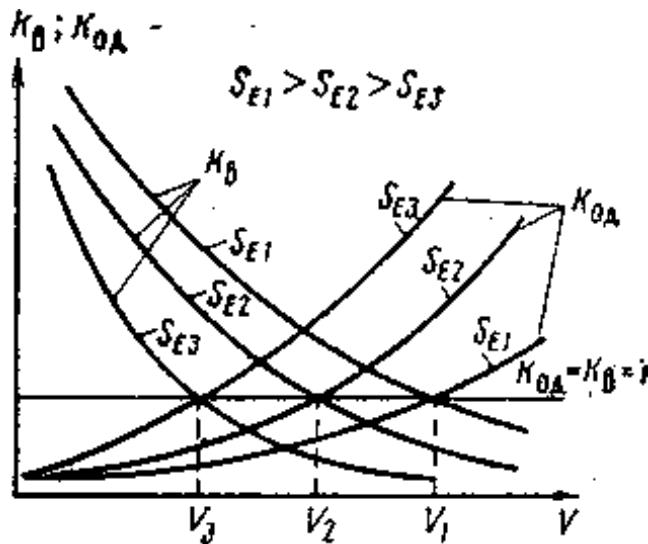
Рис. 8.2. Зависимость коэффициентов видимости K_v и опасности движения K_{од} от скорости: S_{E1} , S_{E2} , S_{E3} — различные значения дальности видимости.
