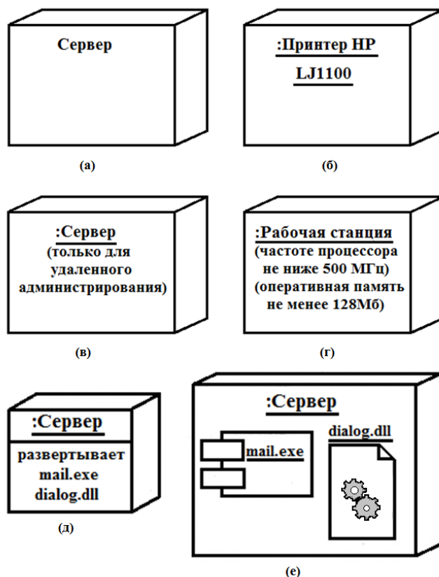
Рис. 4.10. Графические изображения узлов на диаграммах развертывания
