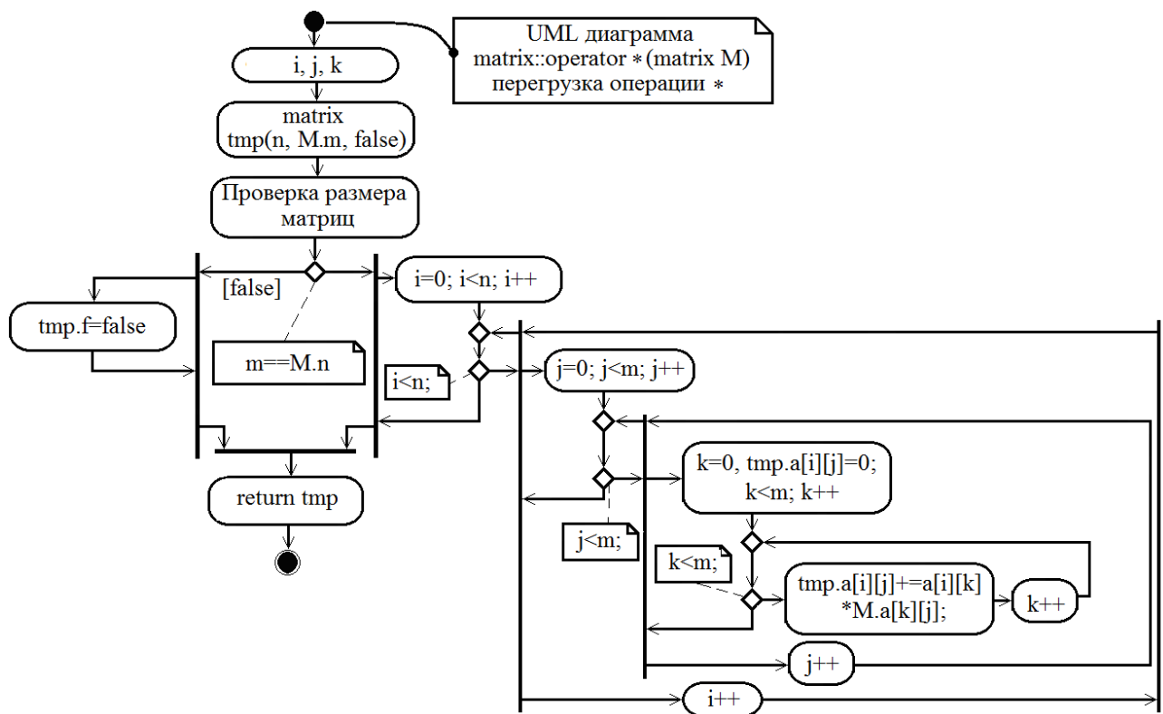
Рис. 6.29. UML – диаграмма для пергрузки операции умножения двух массивов в классе matrix.
