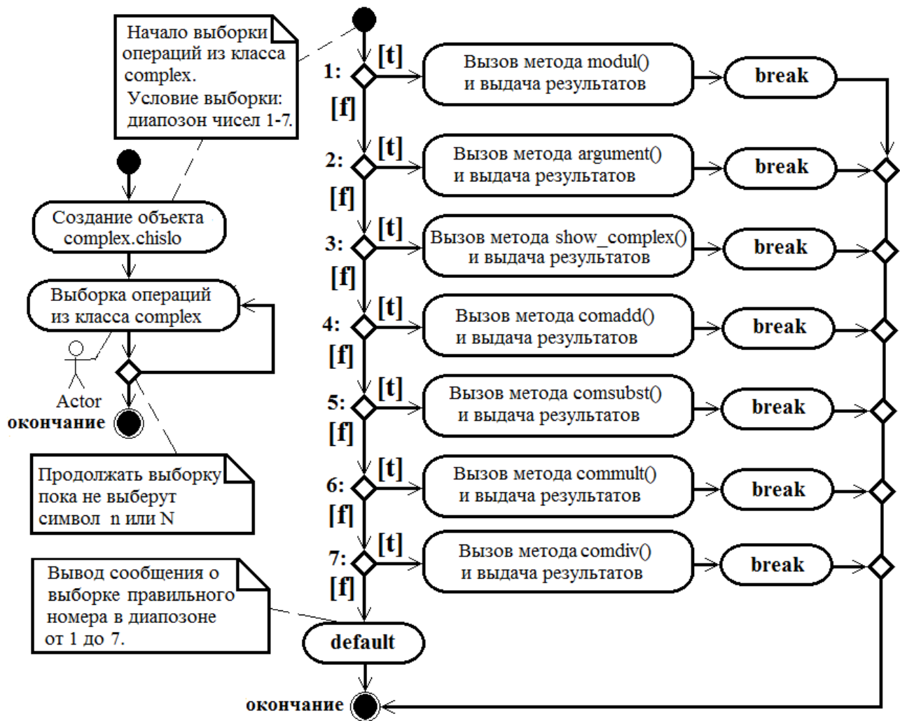
Рис. 6.6. Диаграмма деятельности (UML) для задачи 6.3.
