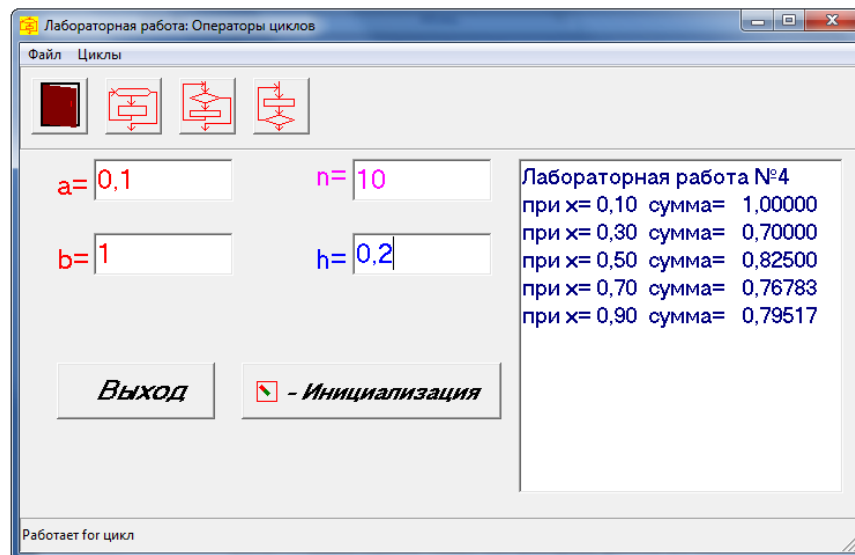
Рис. 4.31. Экспериментальный пример
