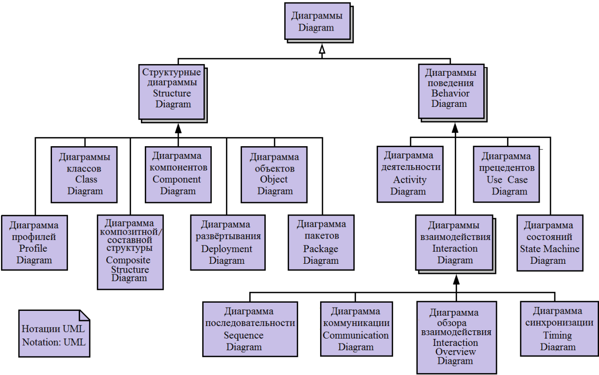
Рис. 3.4. Структура диаграмм.
