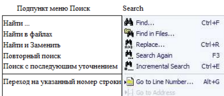
Рис. 1.7. Поисковые операции.
