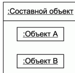
Рис. 4.15. Графическое изображение составного объекта.
