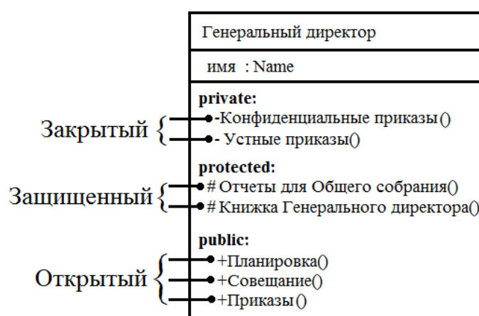
Рис. 4.8. Пример обозначения компонентов в UML диаграммах.
