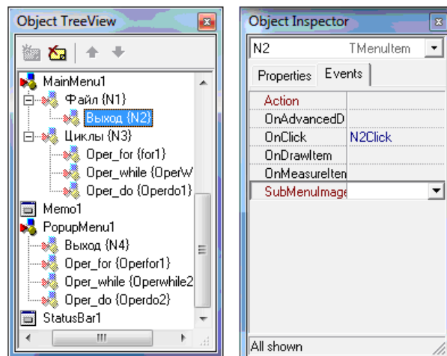
Рис. 4.28. Взаимосвязь функции N2Click с подпунктом меню Выход.
