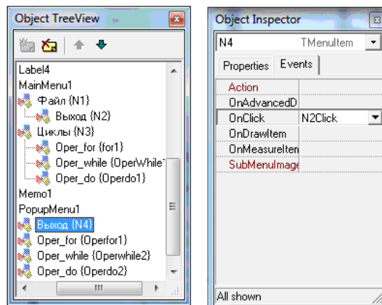
Рис. 4.29. Привязка подпункта «Выход» контекстного меню к функции N2Click в событиях (Events) окна Object Inspector к пункту OnClick.
