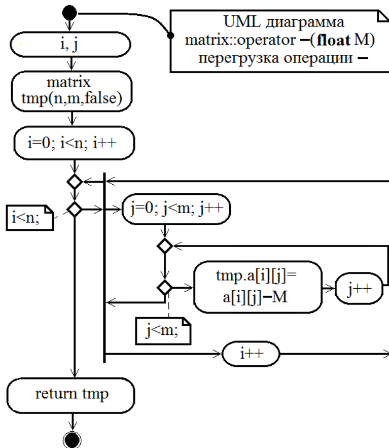
Рис. 6.28. UML –диаграмма, для пергрузки операции вычитания - вещественного числа от массива в классе matrix.
