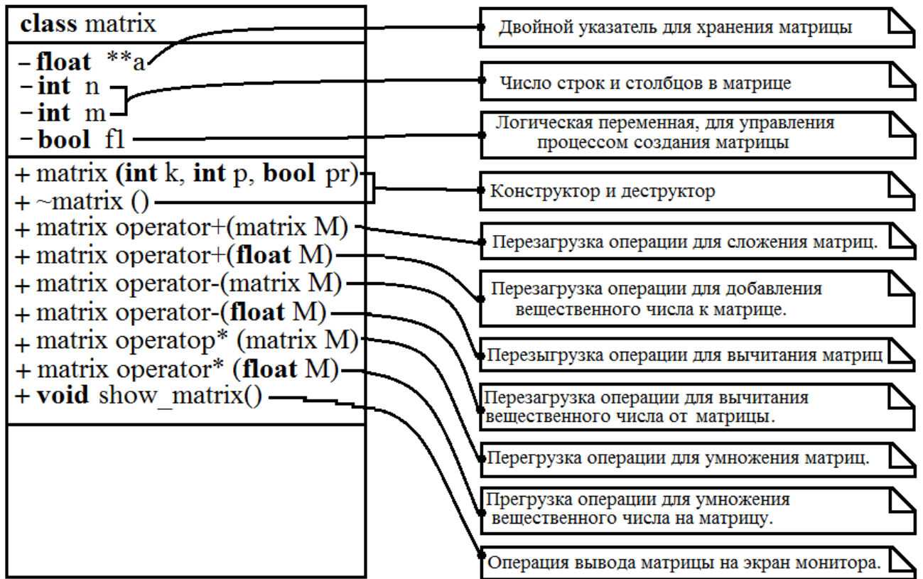
Рис.6.22. Класс matrix .
