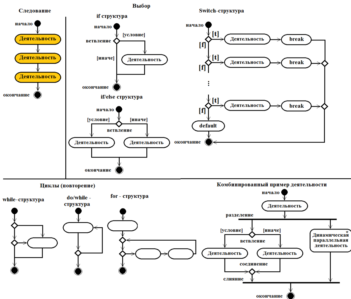
Рис. 3.7. Диаграмма деятельности.
