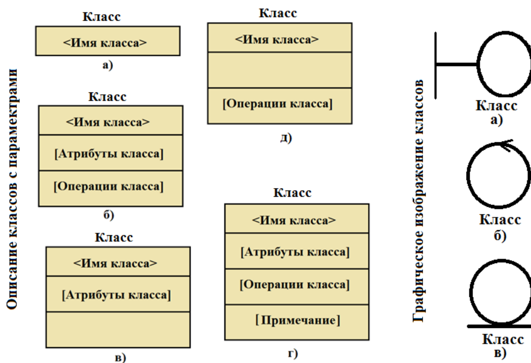
Рис. 3.5. Диаграммы класса.
