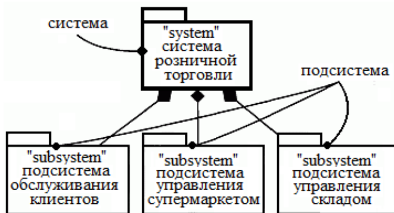
Рис. 4.17. Системы и подсистемы.
